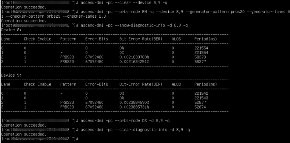
图 8-9 自定义打流示例
