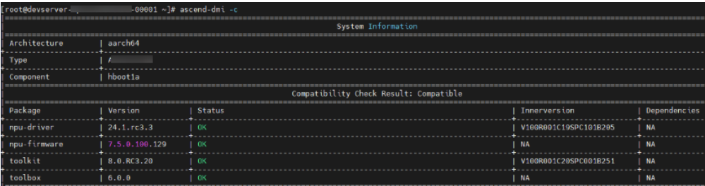
图 8-10 软硬件版本兼容性测试示例
